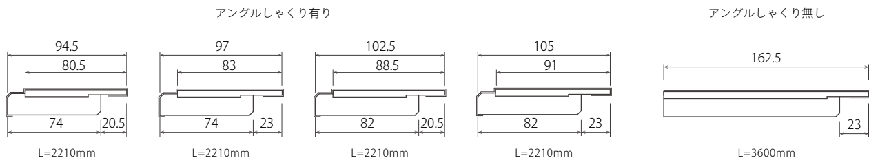
縦断面図 [四方枠]
