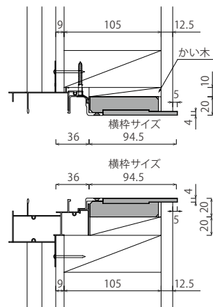
縦断面図 [四方枠]
