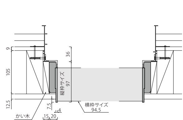
横断面図
